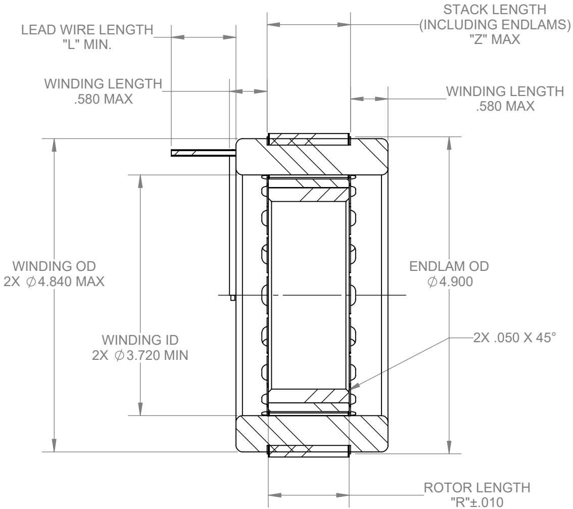
SECTION A-A SCALE 1 : 1.5
